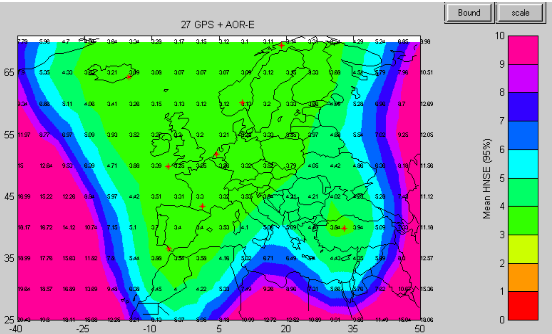
ESTB: Horizontal Accuracy Prediction 27 GPS, SA off
